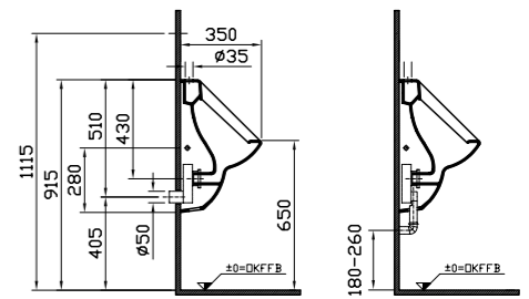
Urinal mit Zulauf oben, Abgang universal Art.-Nr. 6563B0xx-D0202
