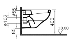
Tiefspül-WC kurze Ausladung, Art.-Nr. 6105L0xx-0075
