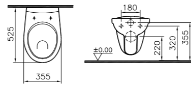
Flachspül-WC, Art.-Nr. 5091L0xx-0075
