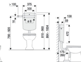
TOPARA 6-9 I-Spülkasten mit definierter 2-Mengen-Spültech- nik und Start-Stopp-Funktion
