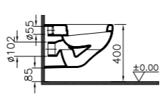
Flachspül-WC kurze Ausladung, Art.-Nr. 6104L0xx-0075
