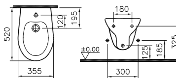
Bidet, Art.-Nr. 6231L0xx-0290
