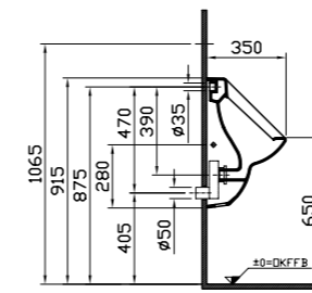
Urinal mit Zulauf hinten, Abgang universal Art.-Nr. 6663B0xx-D0201
