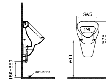
Urinal mit Zulauf hinten, Abgang universal Art.-Nr. 6663B0xx-D0201
