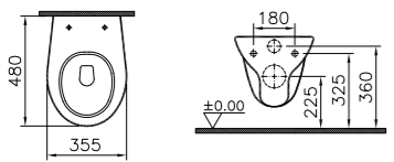
Tiefspül-WC kurze Ausladung, Art.-Nr. 6105L0xx-0075
