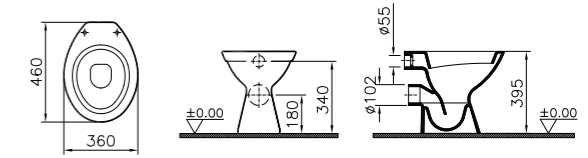
Tiefspül-WC mit waagrechtm Abgang Art.-Nr. 6858L0xx-0101
