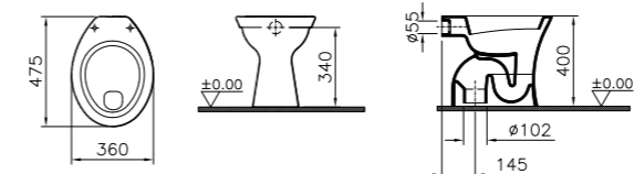
Flachspül-WC mit senkrechtm Abgang Art.-Nr. 6860L0xx-0075
