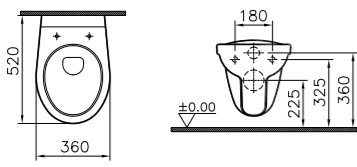
Tiefspül-WC, Art.-Nr. 6855L0xx-0101
