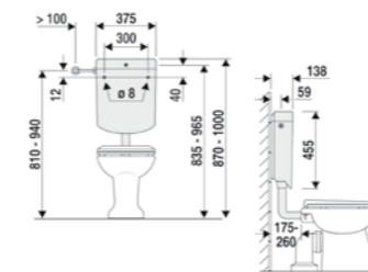
TOPARA 6-9 I-Spülkasten mit Start-Stopp-Technik
