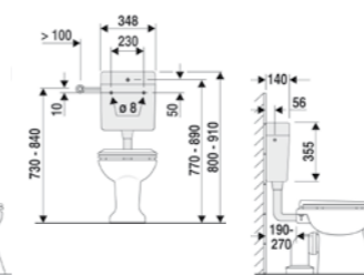
TOPARA 6 I-Spülkasten mit Start-Stopp-Technik
