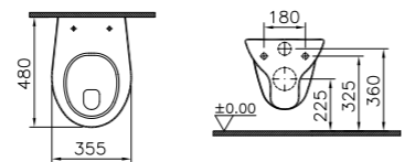
Flachspül-WC kurze Ausladung, Art.-Nr. 6104L0xx-0075
