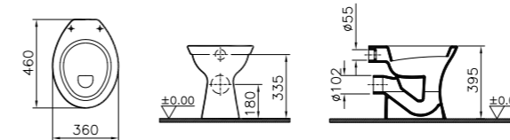
Flachspül-WC mit waagrechtm Abgang Art.-Nr. 6888L0xx-0075
