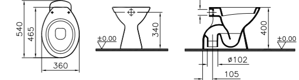
Tiefspül-WC mit senkrechtm Abgang Art.-Nr. 6859L0xx-0075
