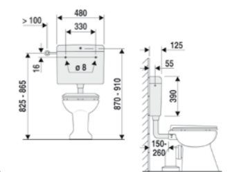
TOPARA 330, 6-9 I Spülkasten mit Start-Stopp-Technik
